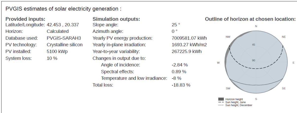
Figura 15 Vlerësimi i energjisë specifike dhe prodhimit të energjisë për 25 - 30 vite
