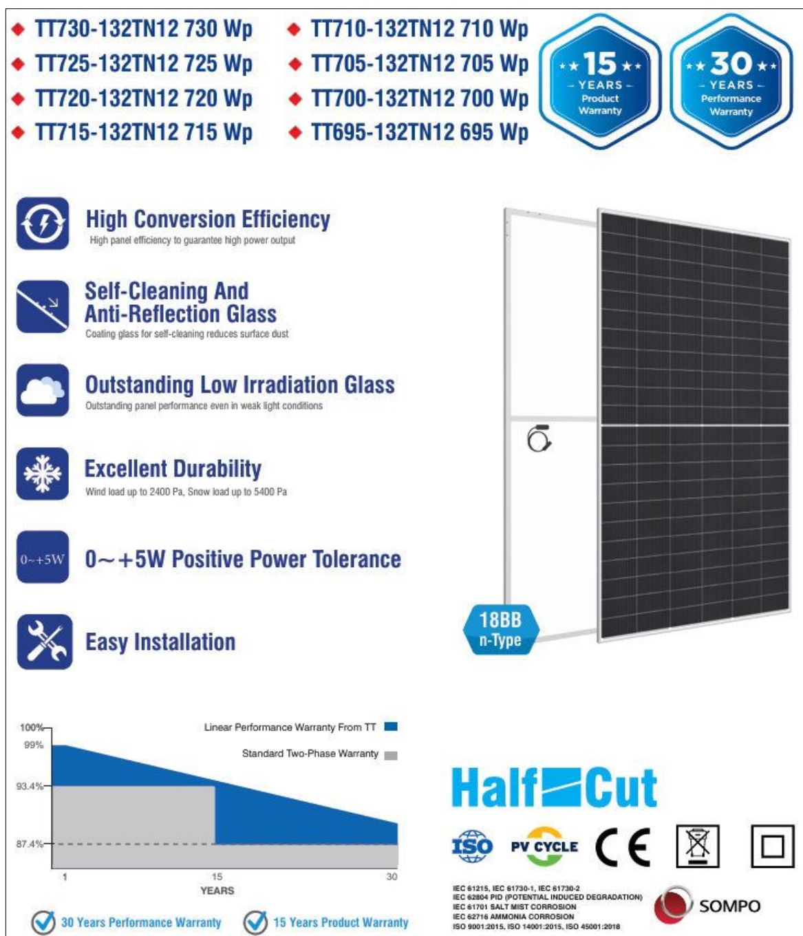
Figura 8 Modeli i Përzgjedhur i panelit solar
