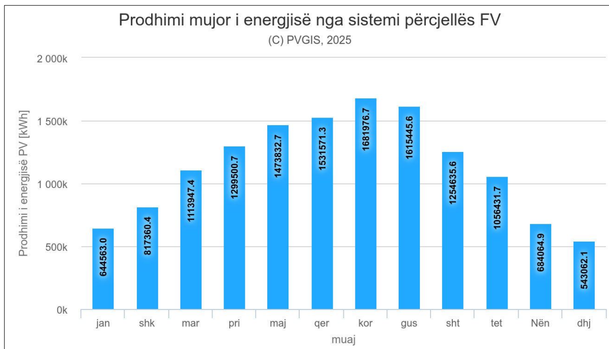
Figura 15 Prodhimi mujor i energjise nga sistemi i parkut solar fotovoltaiak
