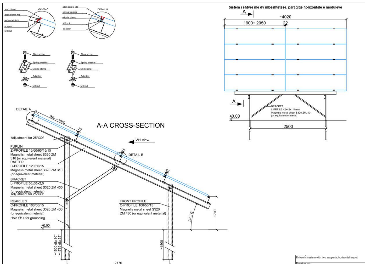
Figura 14 Struktura Fikse e Montimit 4 PANELE OSE 2 PANELE
