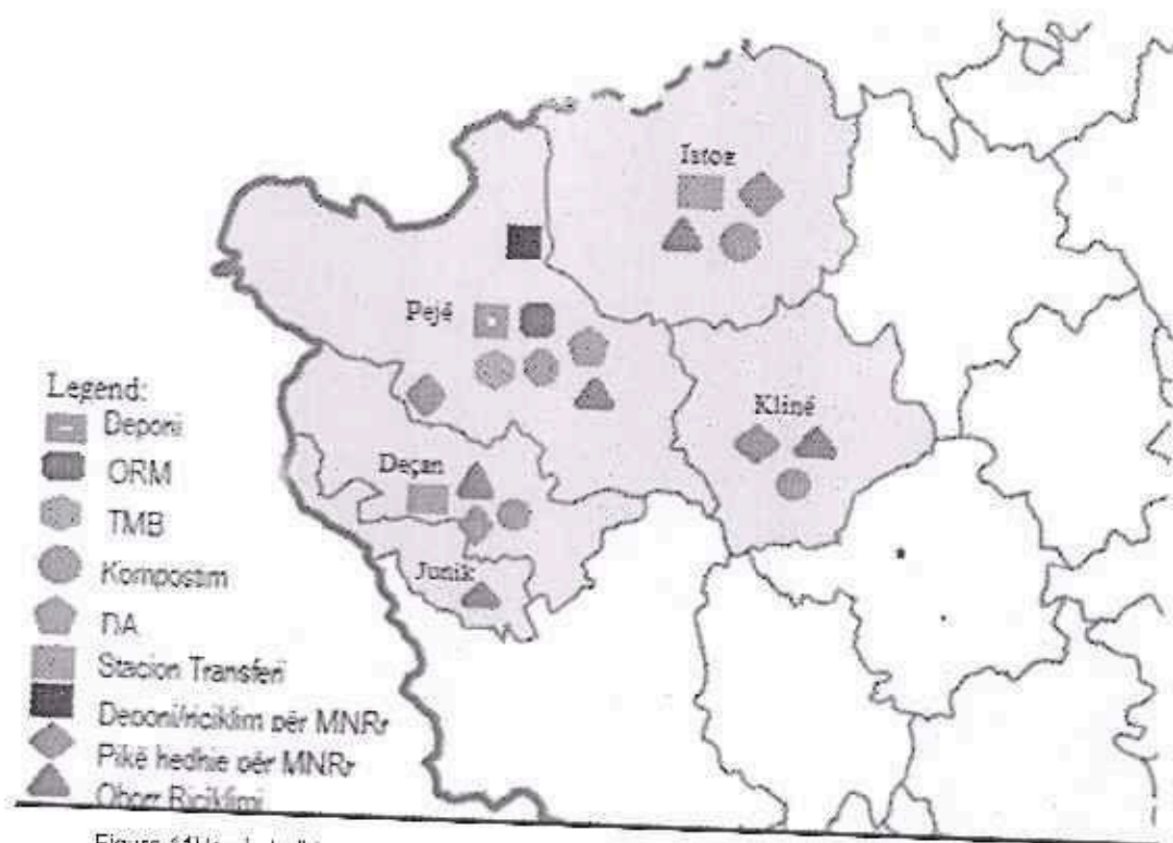
Figura 11 Vëndndodhja e objekteve të parashikuara për menaxhimin e mbeturinave në ZMM 3
